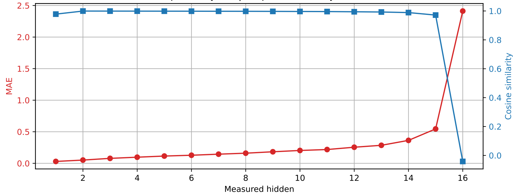
Llama-3.2-1B | Prompt 3 Spared layer 1 | Unquantized vs hybrid
