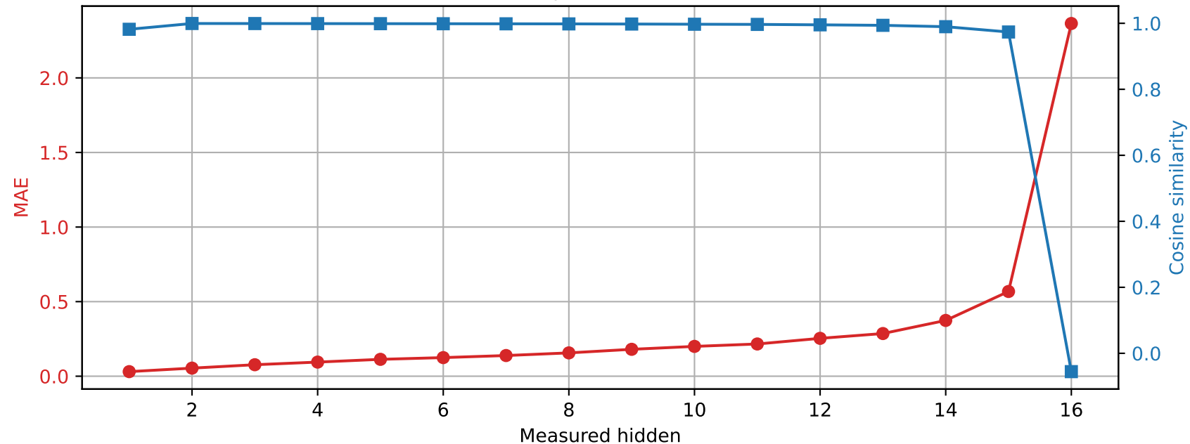
Llama-3.2-1B | Prompt 4 Spared layer 1 | Unquantized vs hybrid
