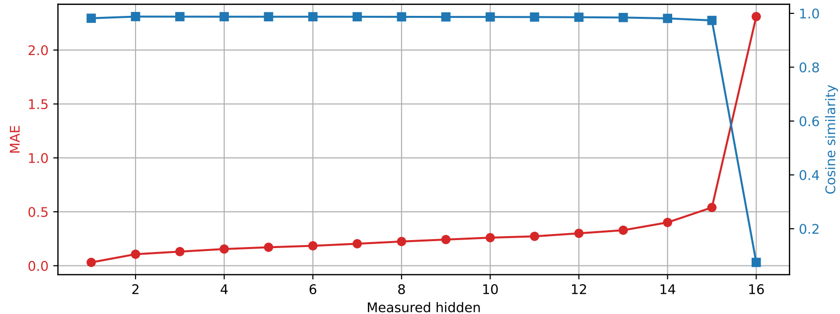
Llama-3.2-1B | Prompt 4 Spared layer 8 | Unquantized vs hybrid
