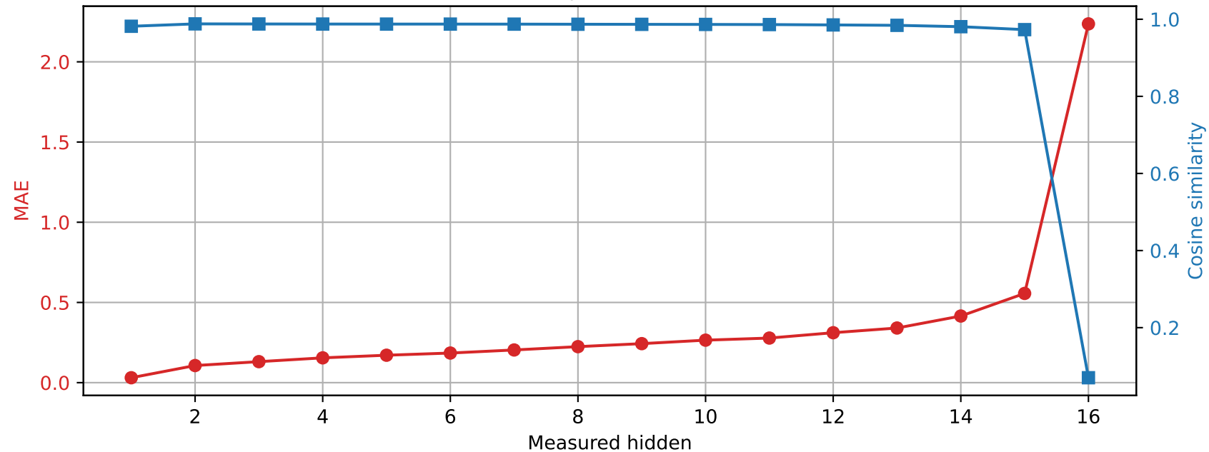
Llama-3.2-1B | Prompt 4 Spared layer 15 | Unquantized vs hybrid
