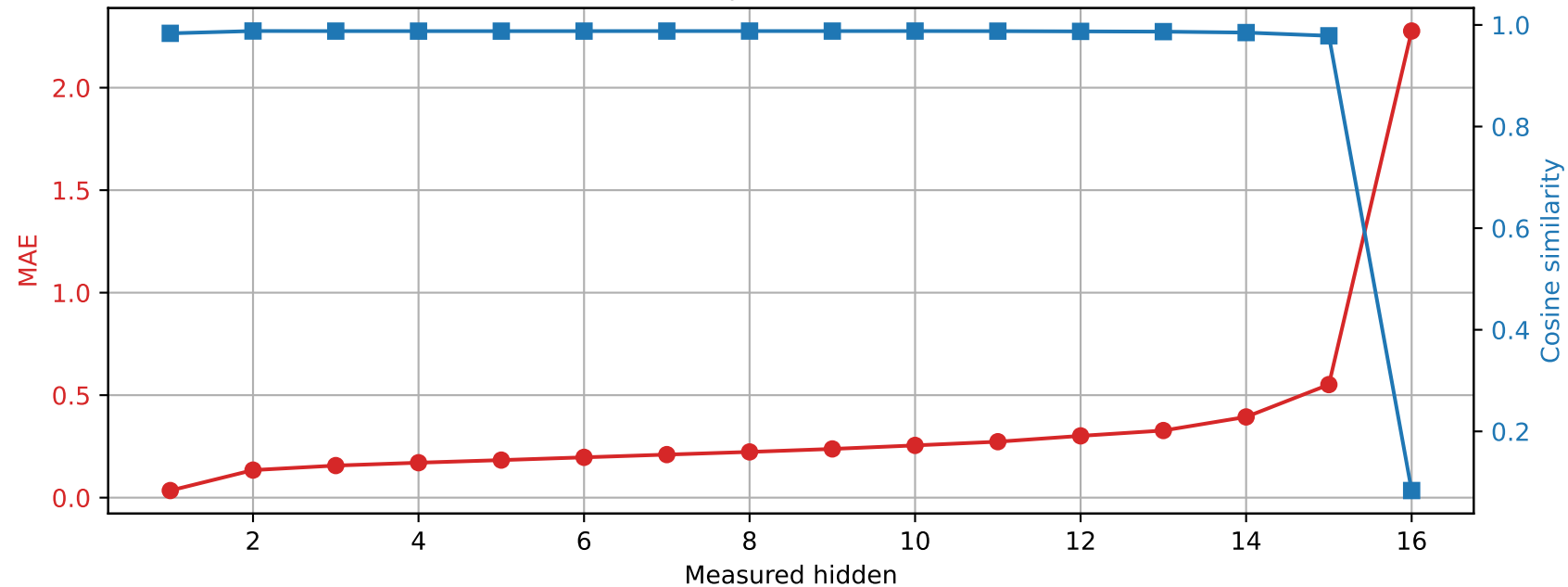
Llama-3.2-1B | Prompt 0 Spared layer 2 | Unquantized vs hybrid
