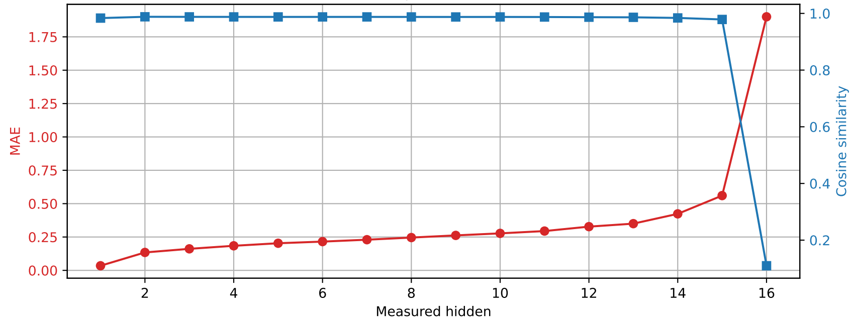
Llama-3.2-1B | Prompt 0 Spared layer 13 | Unquantized vs hybrid
