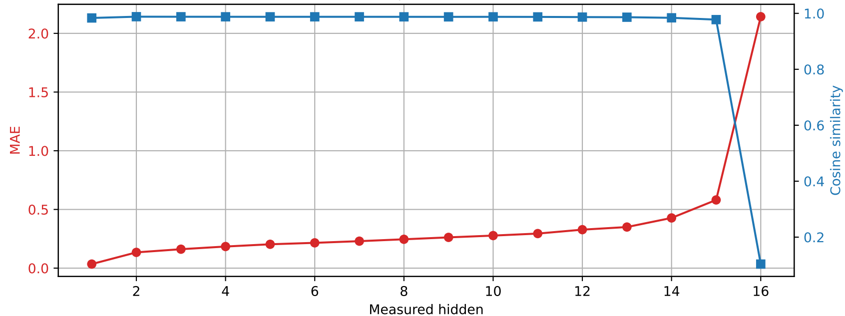
Llama-3.2-1B | Prompt 0 Spared layer 15 | Unquantized vs hybrid
