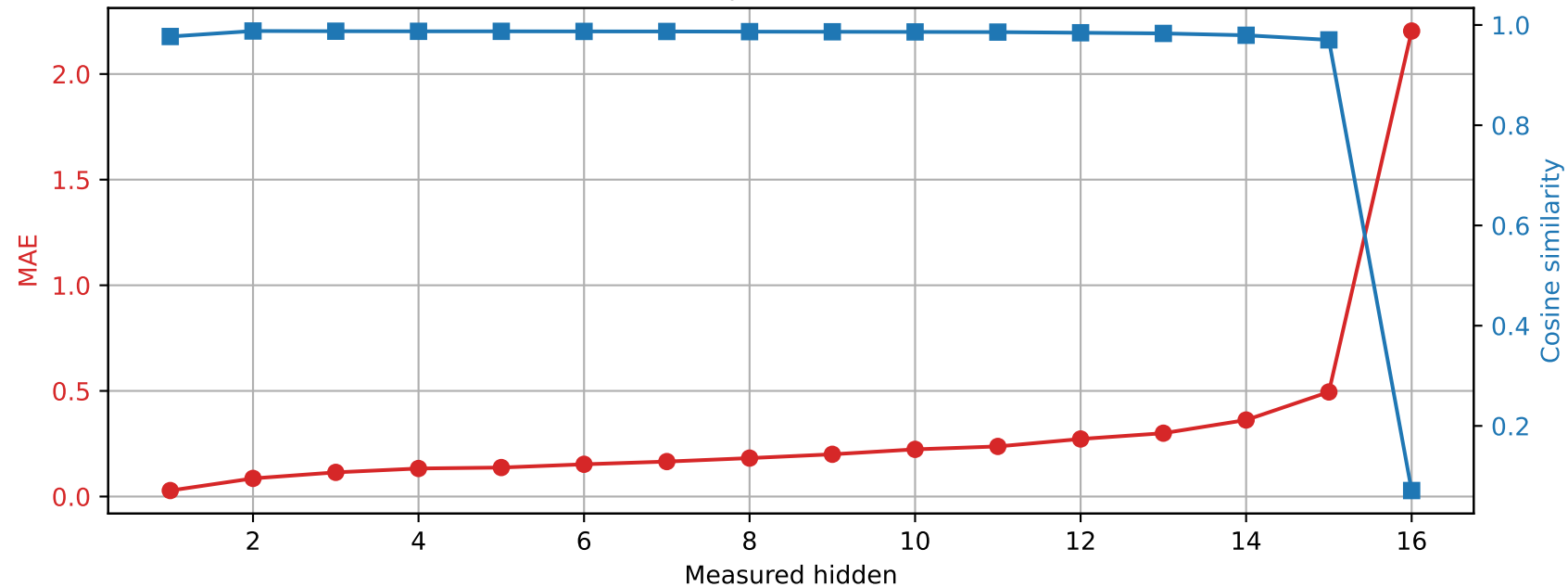
Llama-3.2-1B | Prompt 2 Spared layer 4 | Unquantized vs hybrid
