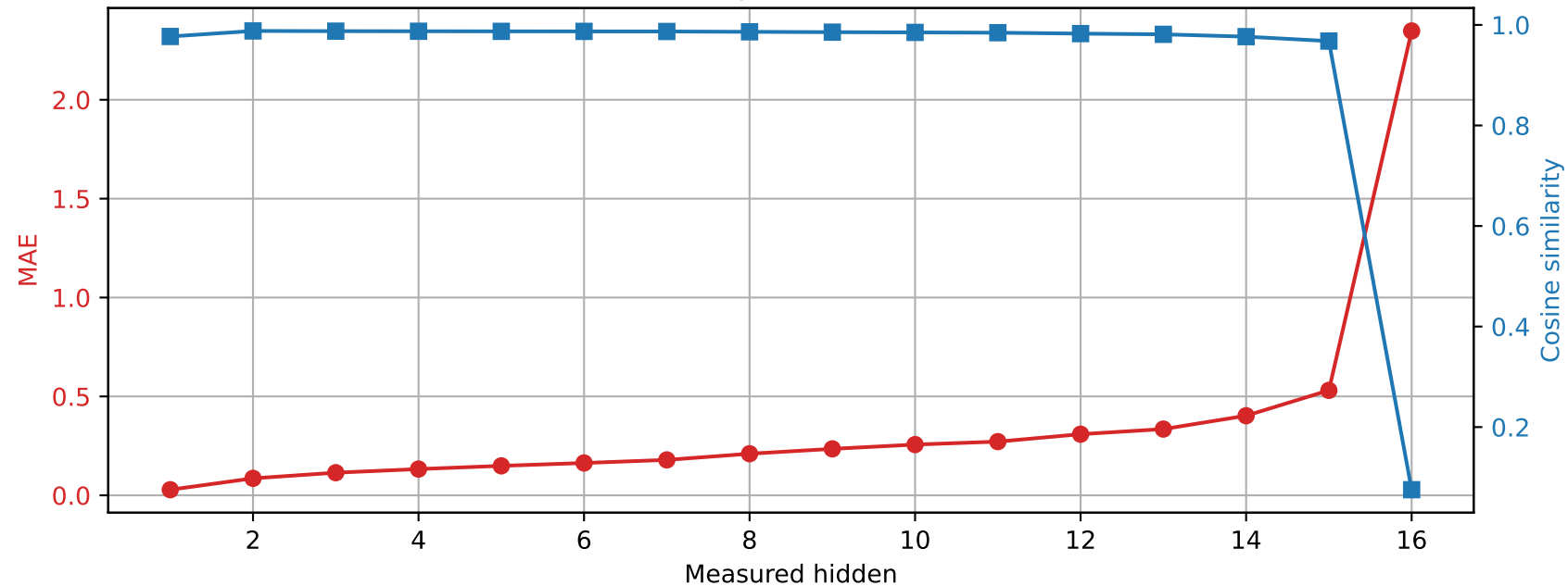
Llama-3.2-1B | Prompt 2 Spared layer 15 | Unquantized vs hybrid
