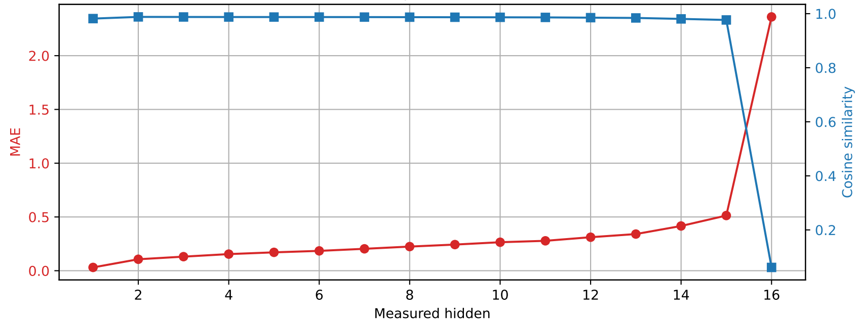
Llama-3.2-1B | Prompt 4 Spared layer 14 | Unquantized vs hybrid
