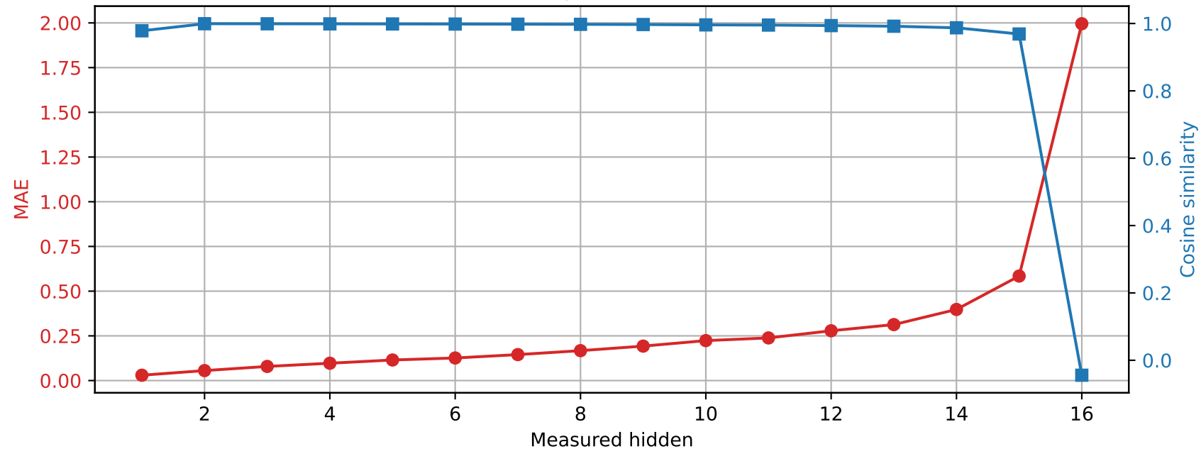
Llama-3.2-1B | Prompt 1 Spared layer 1 | Unquantized vs hybrid
