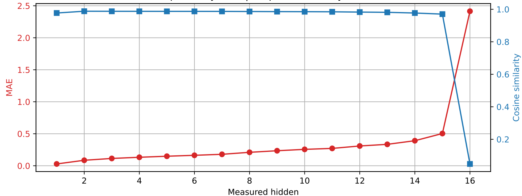
Llama-3.2-1B | Prompt 2 Spared layer 13 | Unquantized vs hybrid
