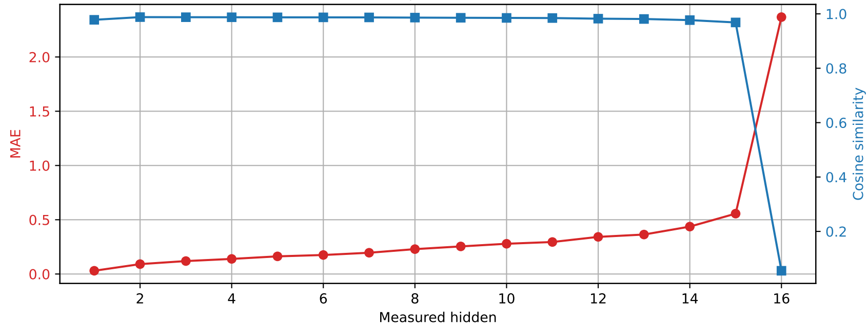
Llama-3.2-1B | Prompt 3 Spared layer 11 | Unquantized vs hybrid
