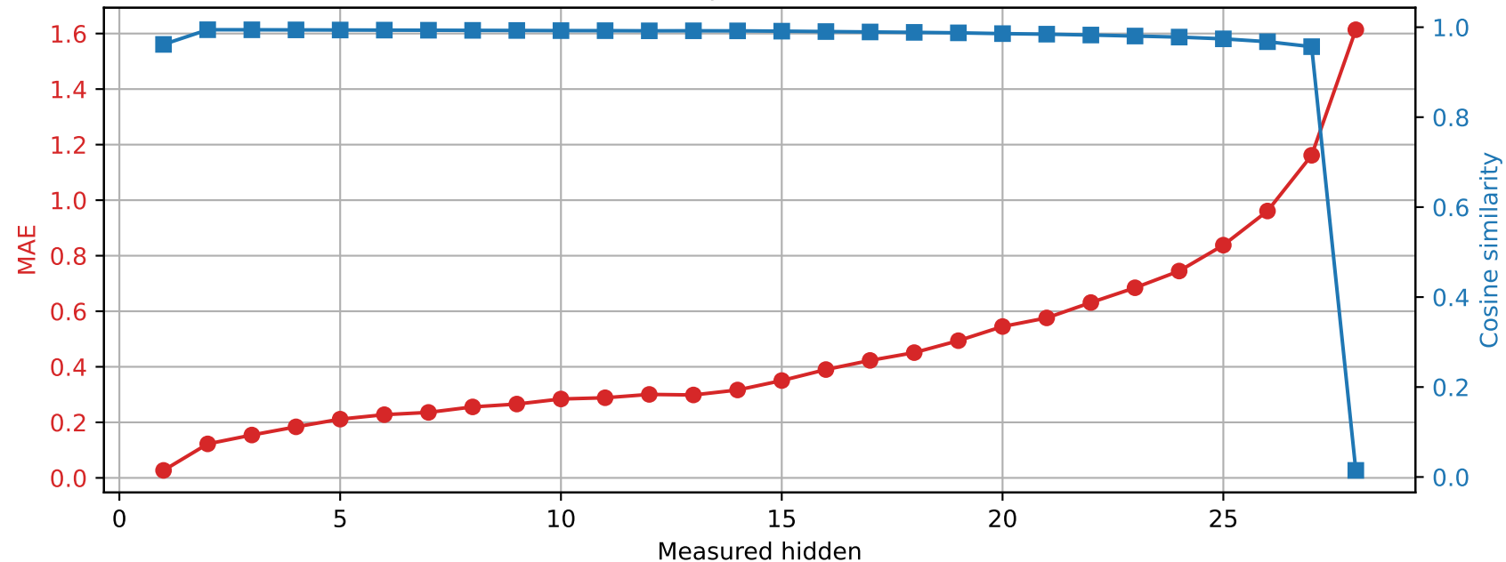
Llama-3.2-3B | Prompt 0 Spared layer 22 | Unquantized vs hybrid
