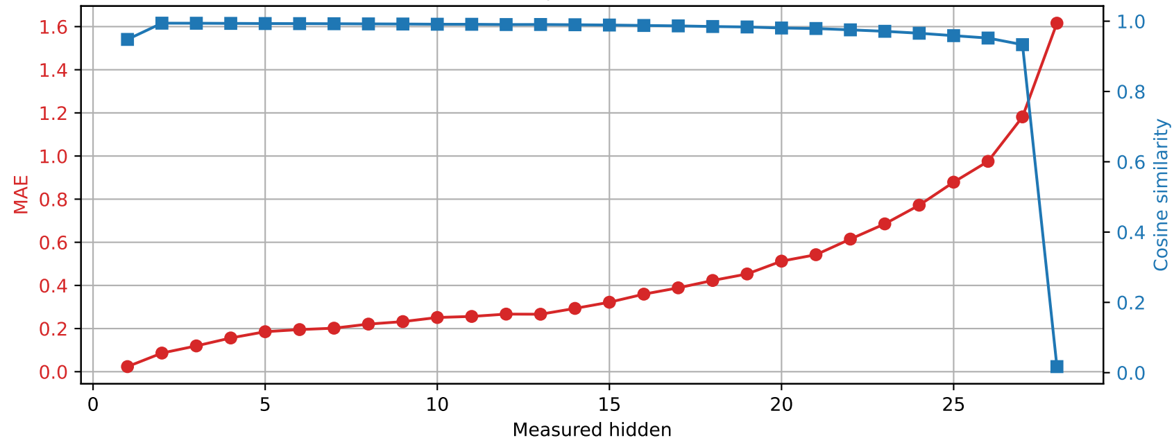
Llama-3.2-3B | Prompt 1 Spared layer 5 | Unquantized vs hybrid
