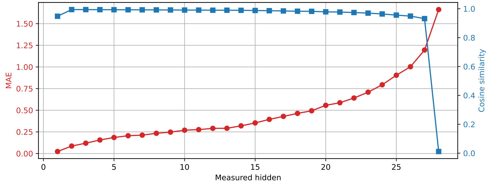
Llama-3.2-3B | Prompt 1 Spared layer 21 | Unquantized vs hybrid
