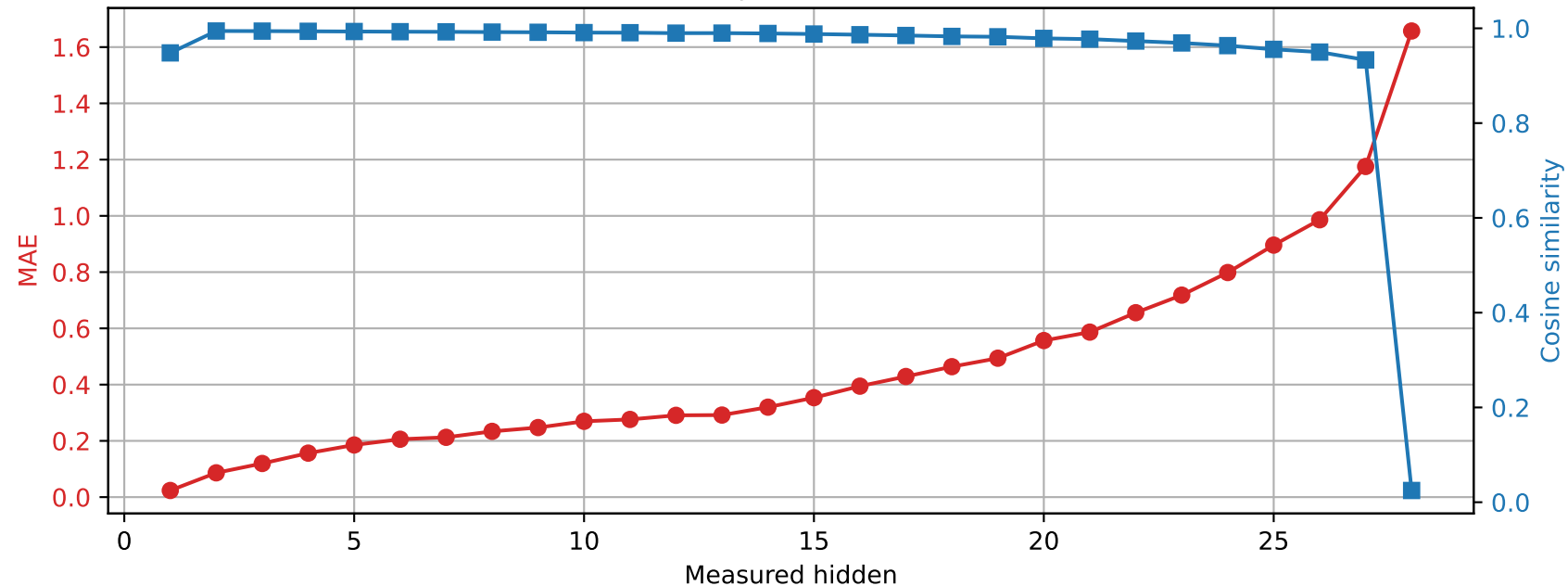
Llama-3.2-3B | Prompt 1 Spared layer 23 | Unquantized vs hybrid
