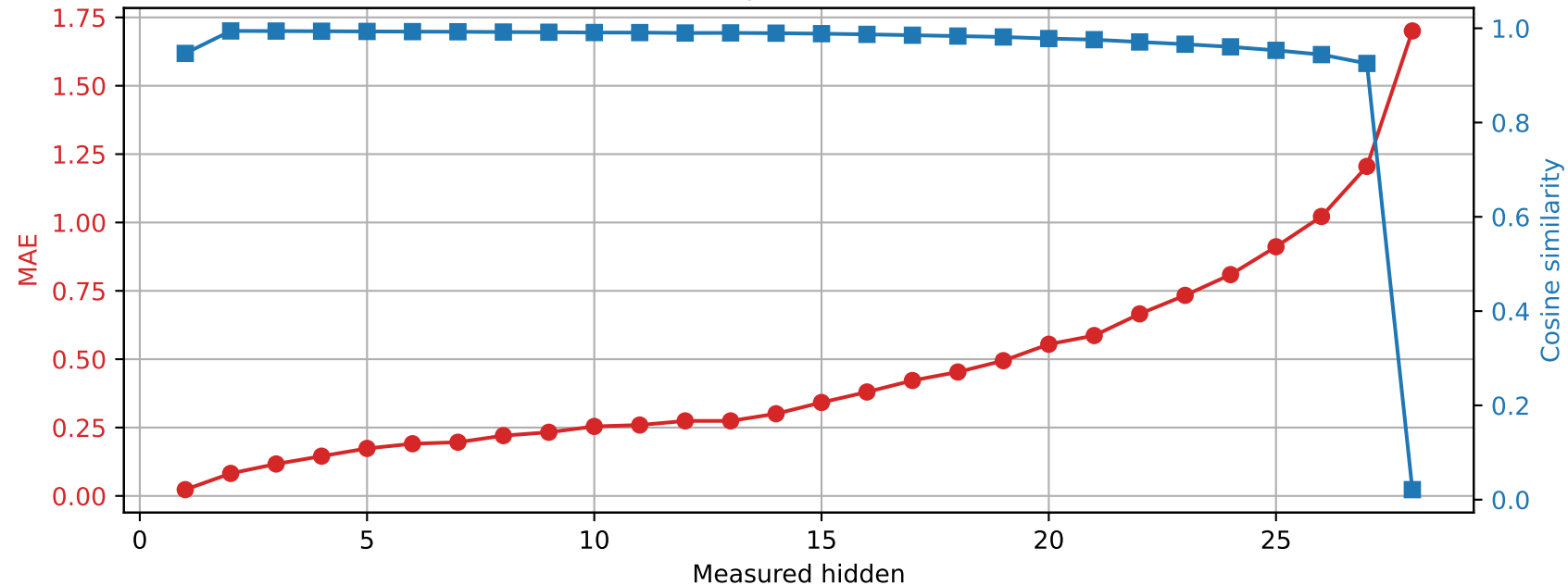
Llama-3.2-3B | Prompt 2 Spared layer 18 | Unquantized vs hybrid
