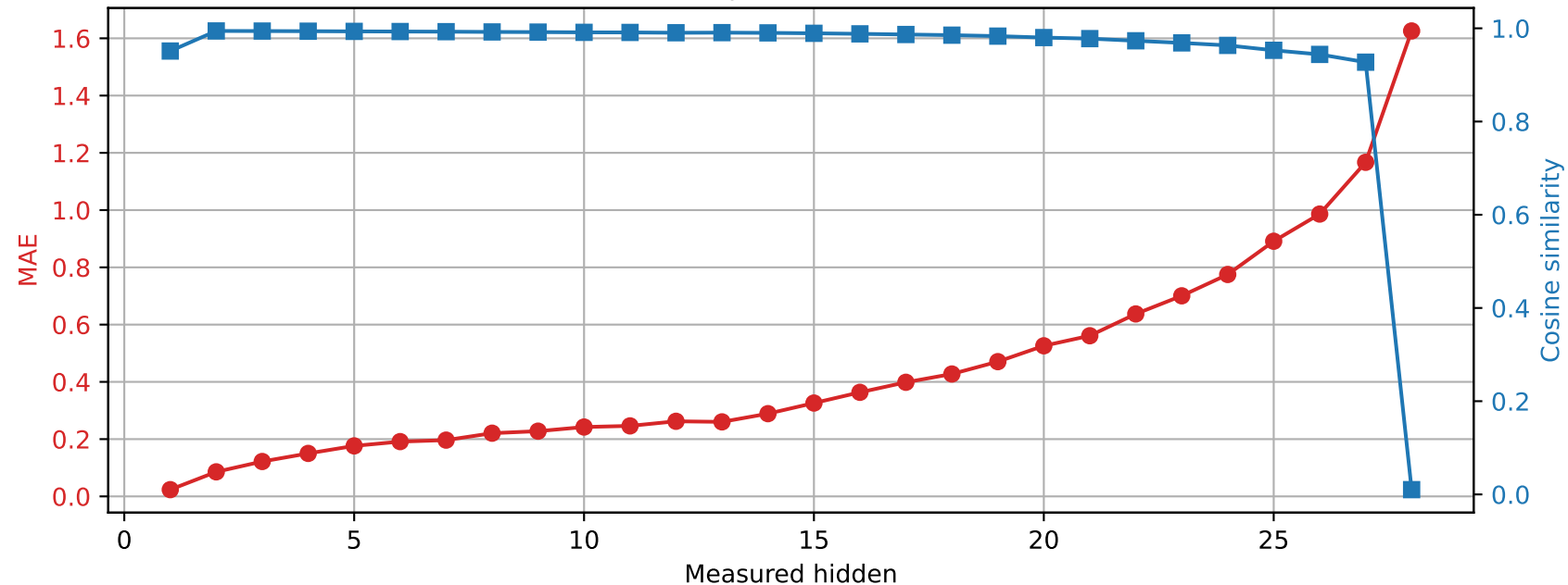
Llama-3.2-3B | Prompt 3 Spared layer 3 | Unquantized vs hybrid
