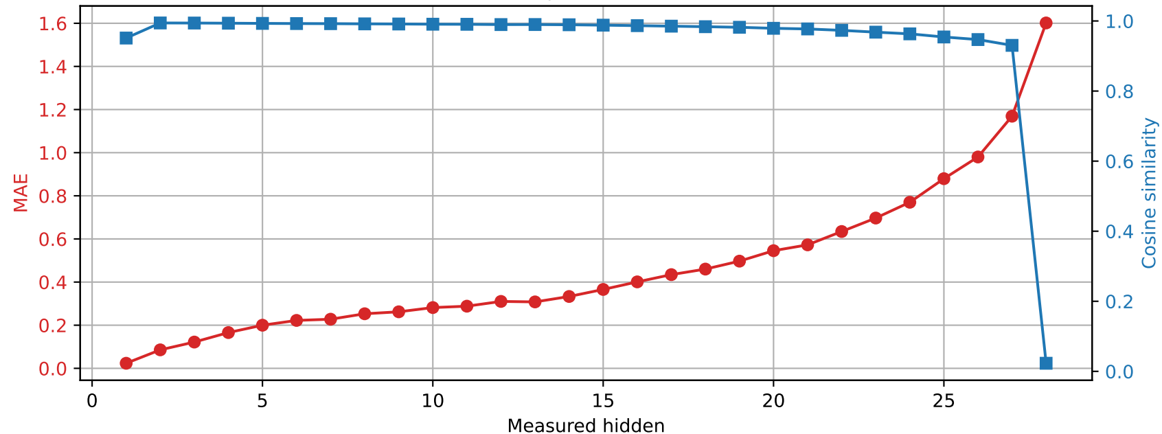
Llama-3.2-3B | Prompt 3 Spared layer 11 | Unquantized vs hybrid
