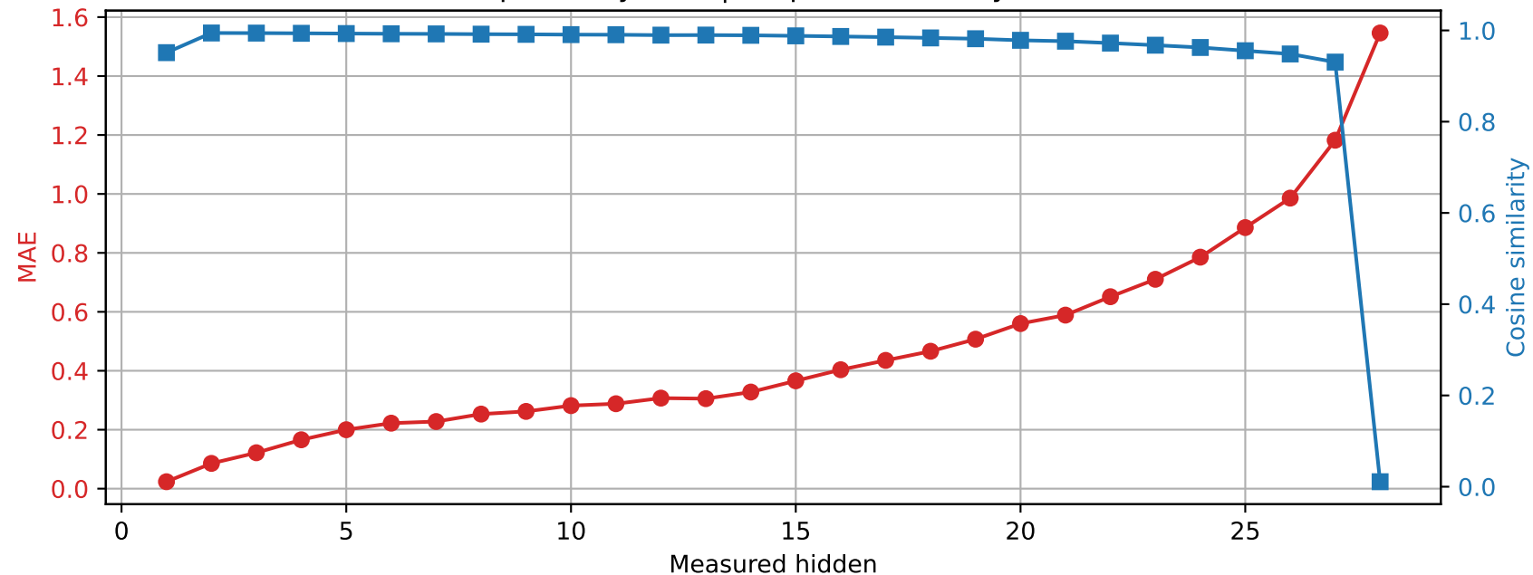
Llama-3.2-3B | Prompt 3 Spared layer 14 | Unquantized vs hybrid
