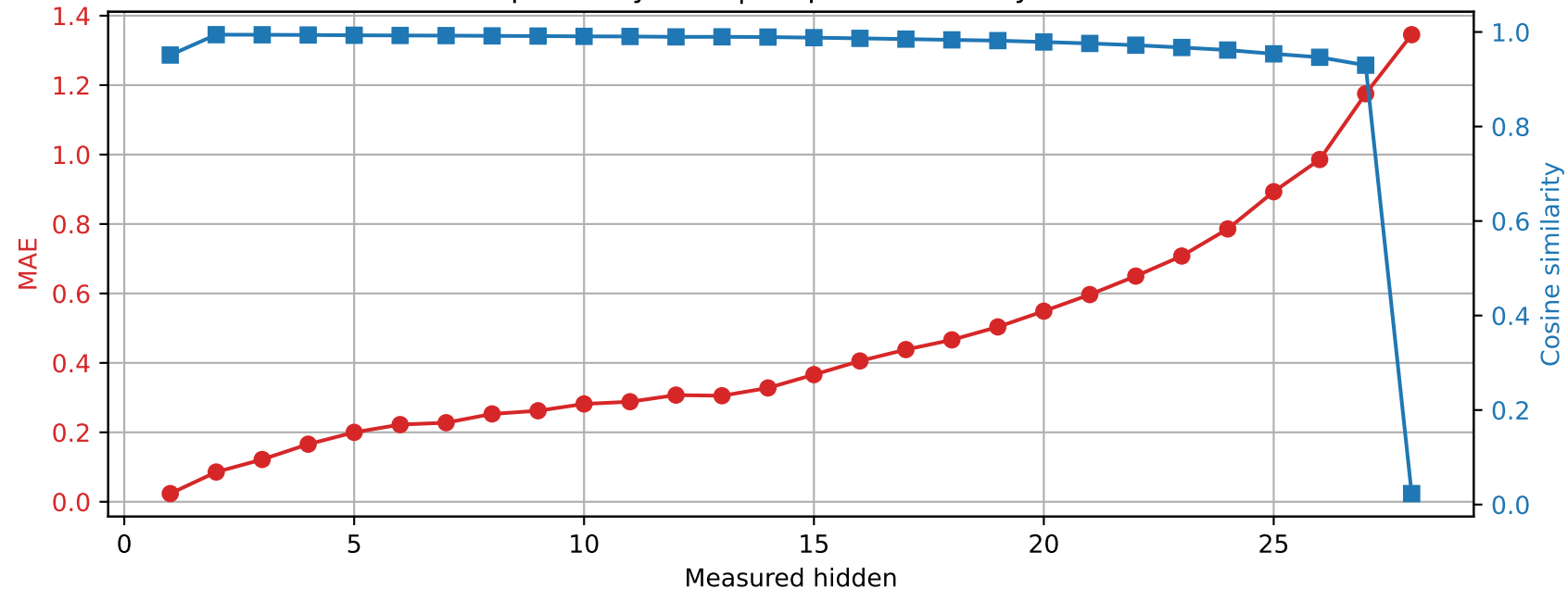
Llama-3.2-3B | Prompt 3 Spared layer 20 | Unquantized vs hybrid
