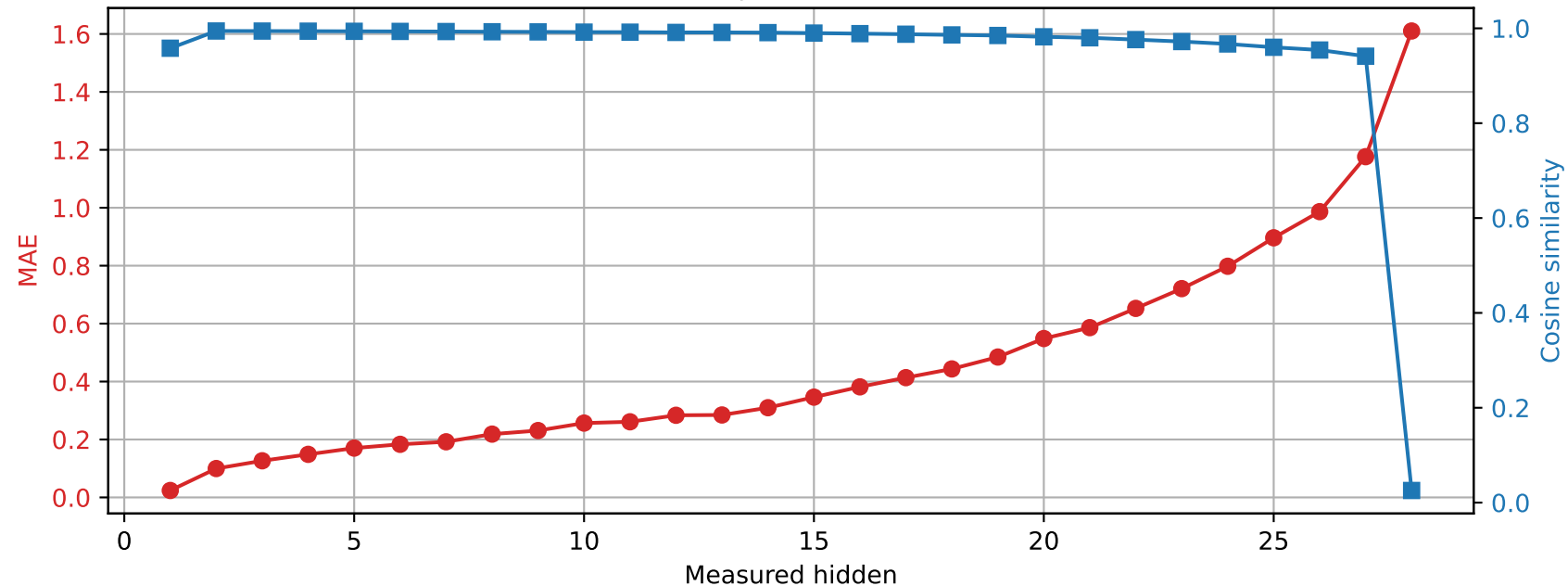
Llama-3.2-3B | Prompt 4 Spared layer 11 | Unquantized vs hybrid
