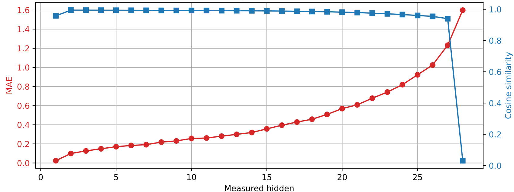
Llama-3.2-3B | Prompt 4 Spared layer 12 | Unquantized vs hybrid
