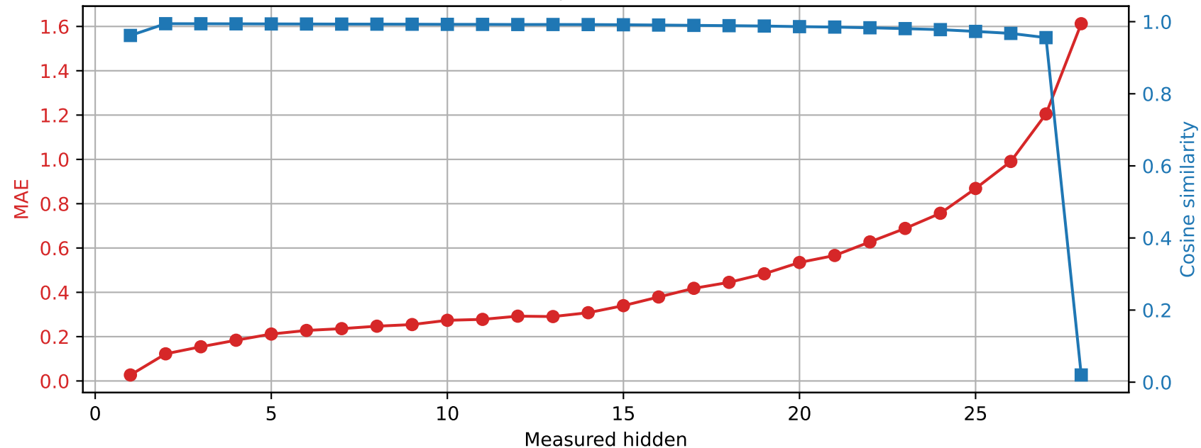
Llama-3.2-3B | Prompt 0 Spared layer 7 | Unquantized vs hybrid
