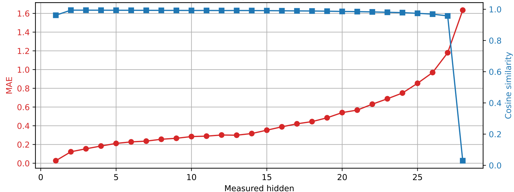
Llama-3.2-3B | Prompt 0 Spared layer 14 | Unquantized vs hybrid
