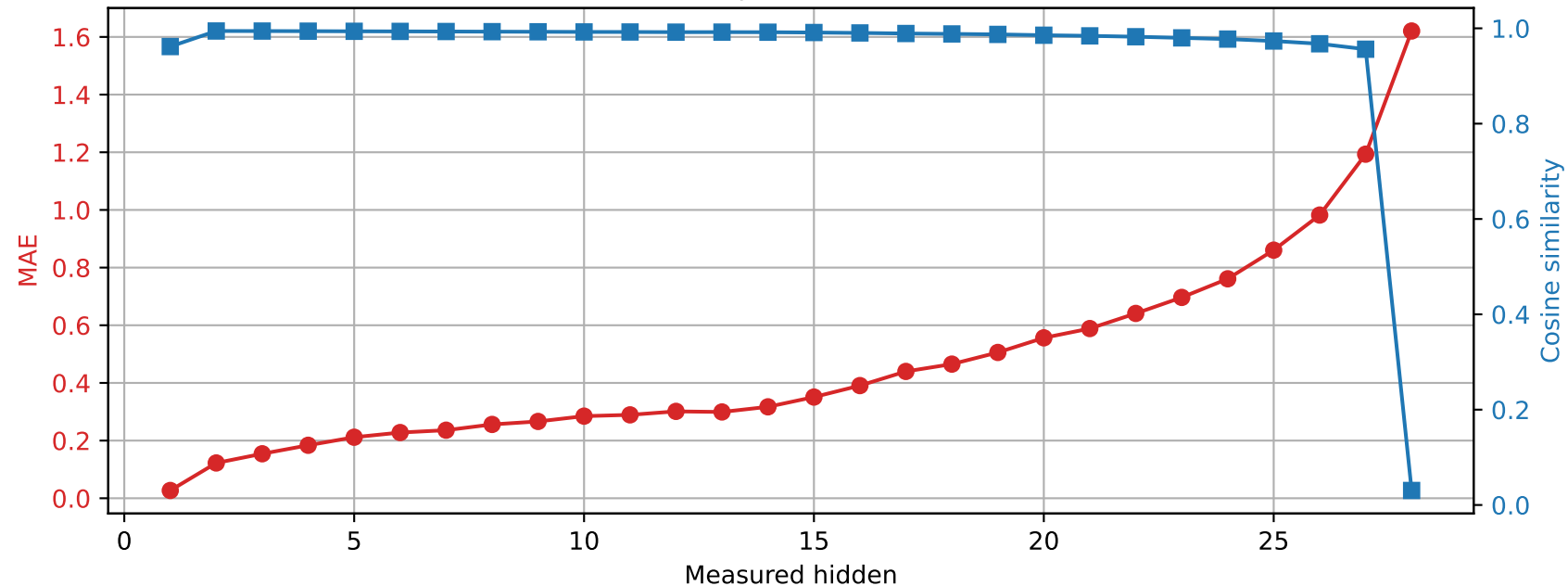
Llama-3.2-3B | Prompt 0 Spared layer 16 | Unquantized vs hybrid
