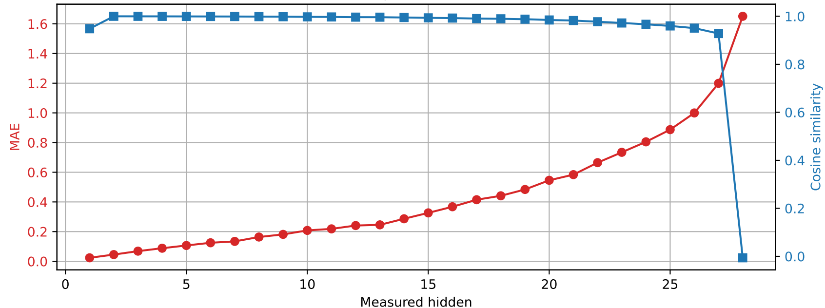
Llama-3.2-3B | Prompt 1 Spared layer 1 | Unquantized vs hybrid
