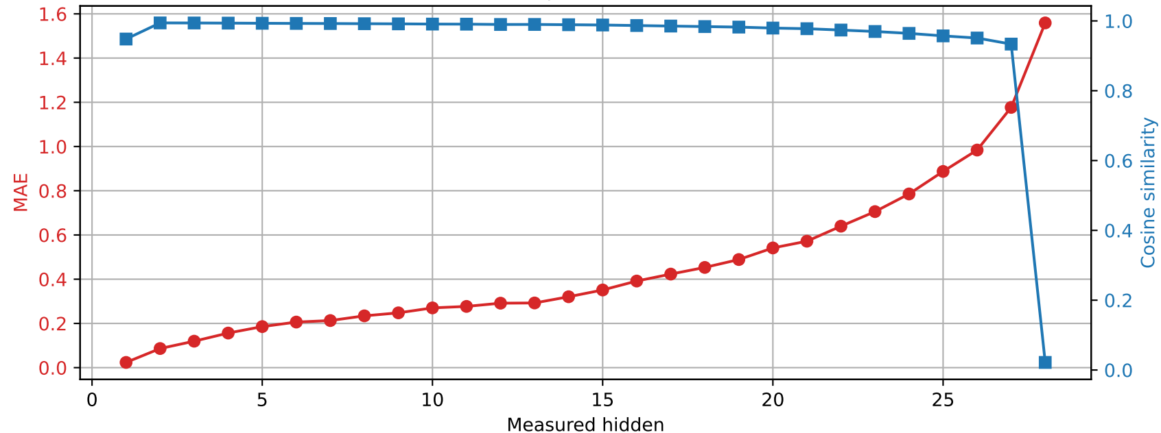
Llama-3.2-3B | Prompt 1 Spared layer 14 | Unquantized vs hybrid
