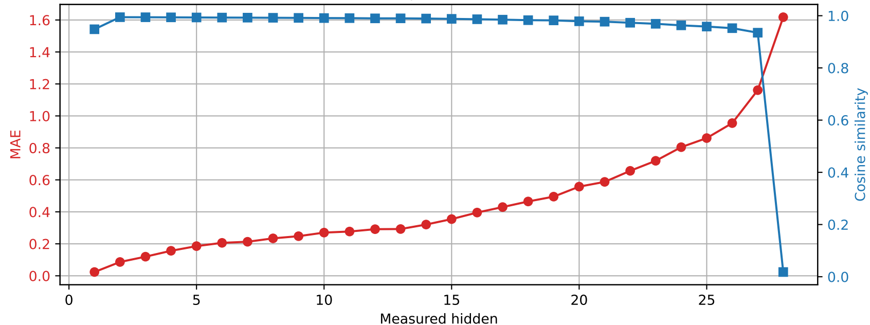
Llama-3.2-3B | Prompt 1 Spared layer 24 | Unquantized vs hybrid
