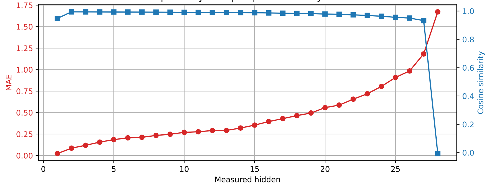
Llama-3.2-3B | Prompt 1 Spared layer 25 | Unquantized vs hybrid
