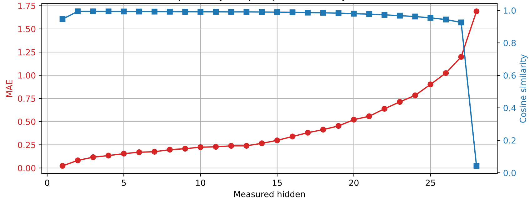
Llama-3.2-3B | Prompt 2 Spared layer 3 | Unquantized vs hybrid
