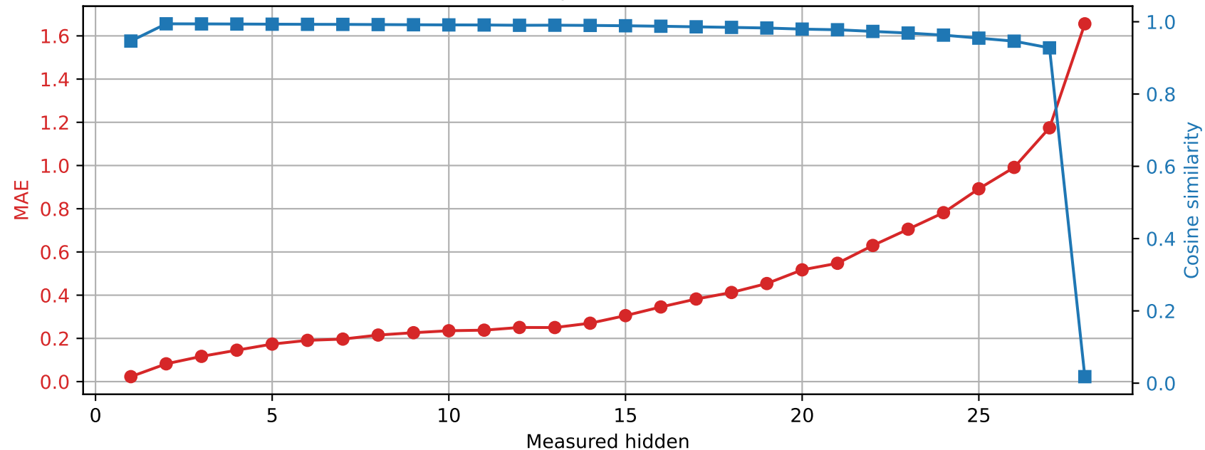
Llama-3.2-3B | Prompt 2 Spared layer 6 | Unquantized vs hybrid
