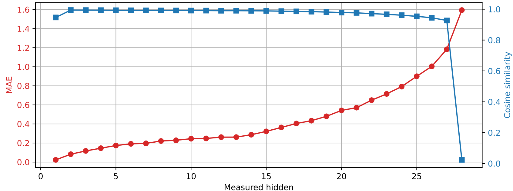
Llama-3.2-3B | Prompt 2 Spared layer 8 | Unquantized vs hybrid
