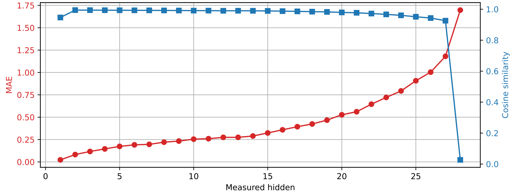
Llama-3.2-3B | Prompt 2 Spared layer 13 | Unquantized vs hybrid
