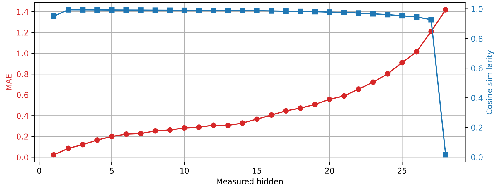
Llama-3.2-3B | Prompt 3 Spared layer 16 | Unquantized vs hybrid
