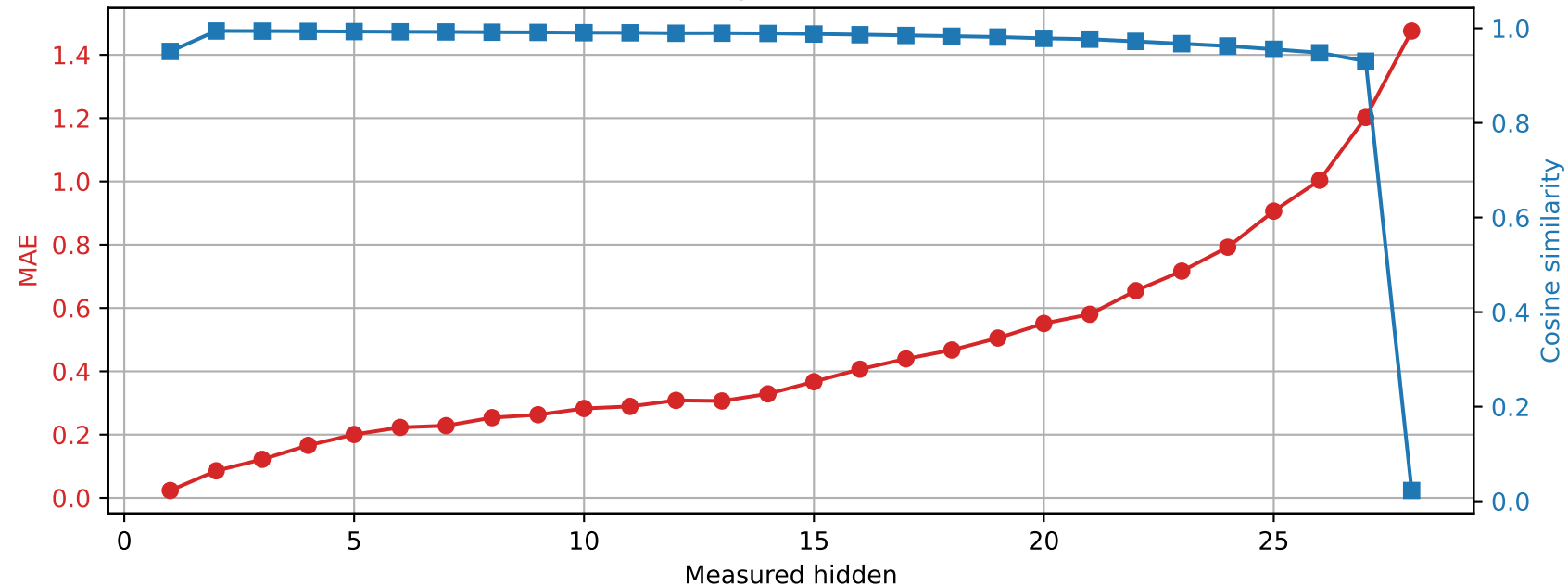
Llama-3.2-3B | Prompt 3 Spared layer 18 | Unquantized vs hybrid
