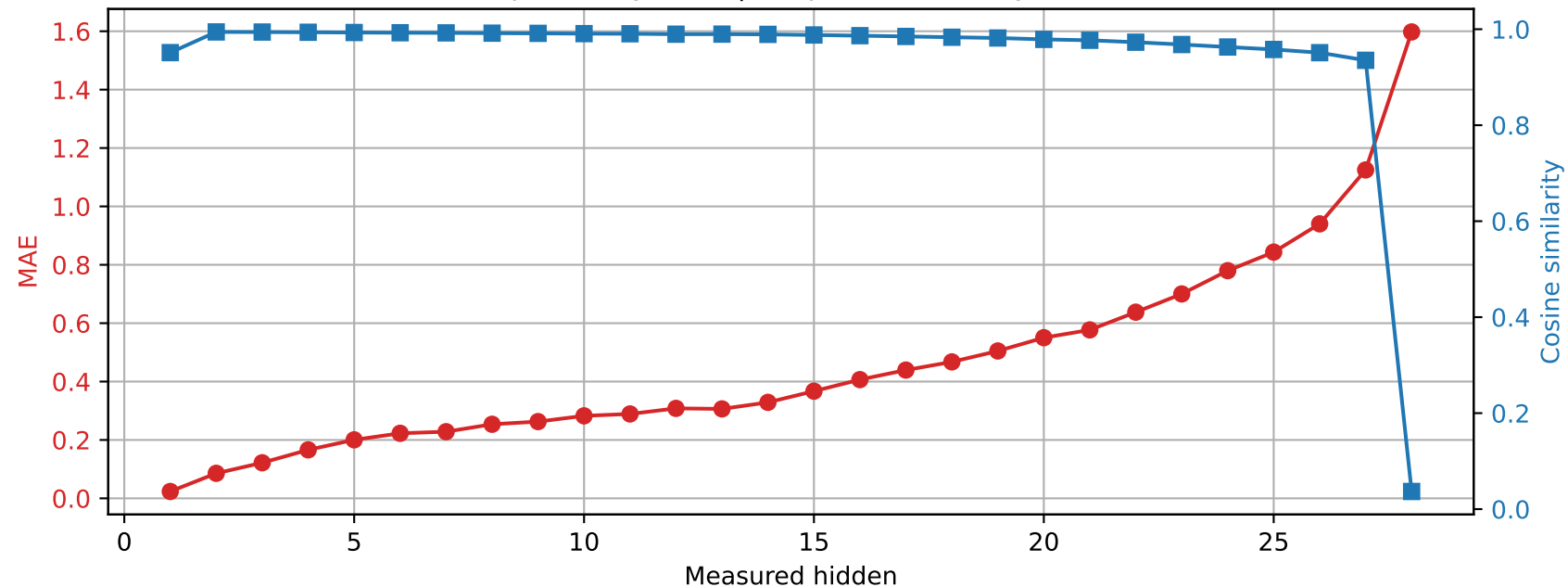
Llama-3.2-3B | Prompt 3 Spared layer 24 | Unquantized vs hybrid
