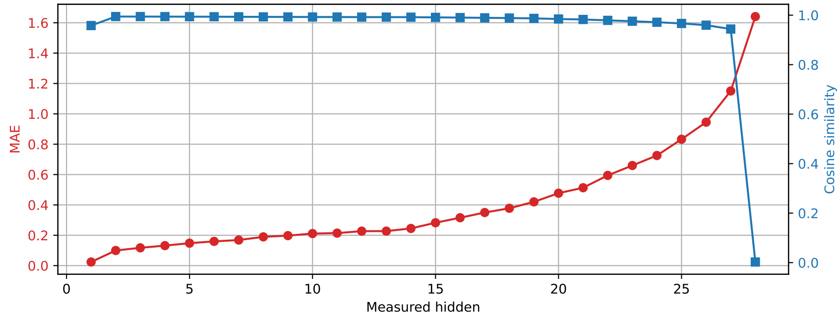
Llama-3.2-3B | Prompt 4 Spared layer 2 | Unquantized vs hybrid
