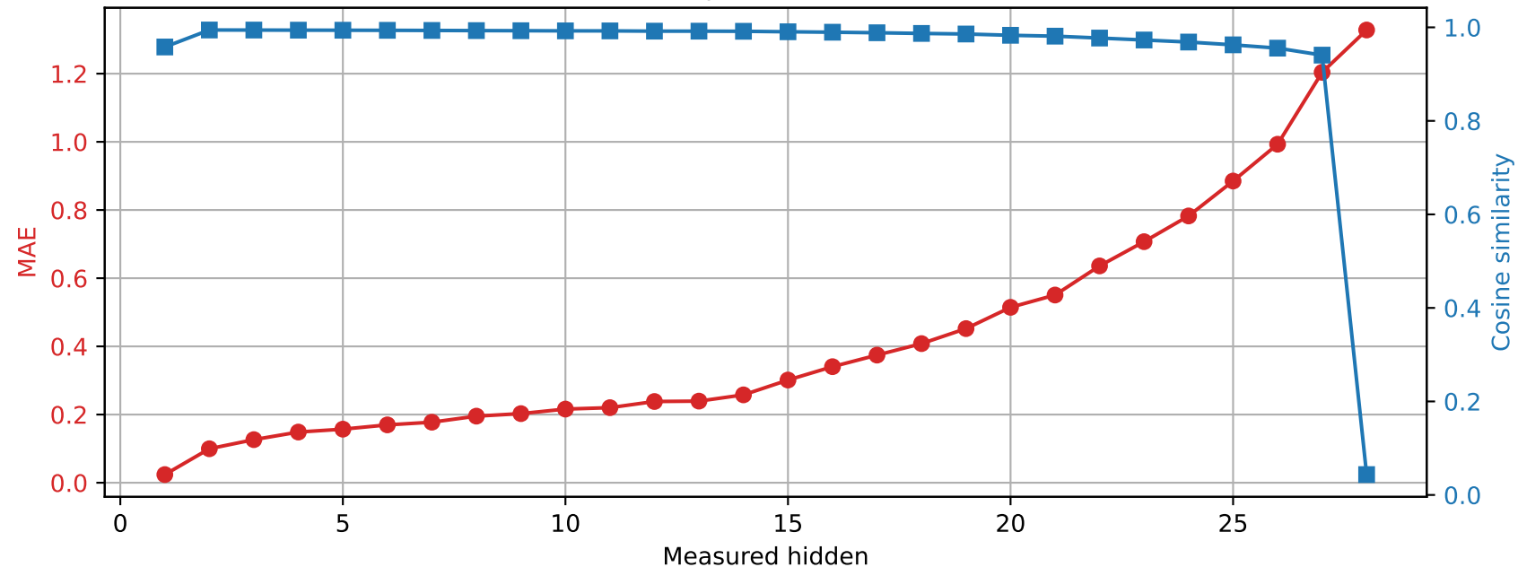
Llama-3.2-3B | Prompt 4 Spared layer 4 | Unquantized vs hybrid
