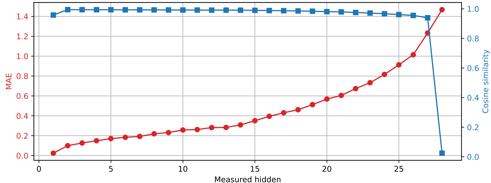
Llama-3.2-3B | Prompt 4 Spared layer 18 | Unquantized vs hybrid
