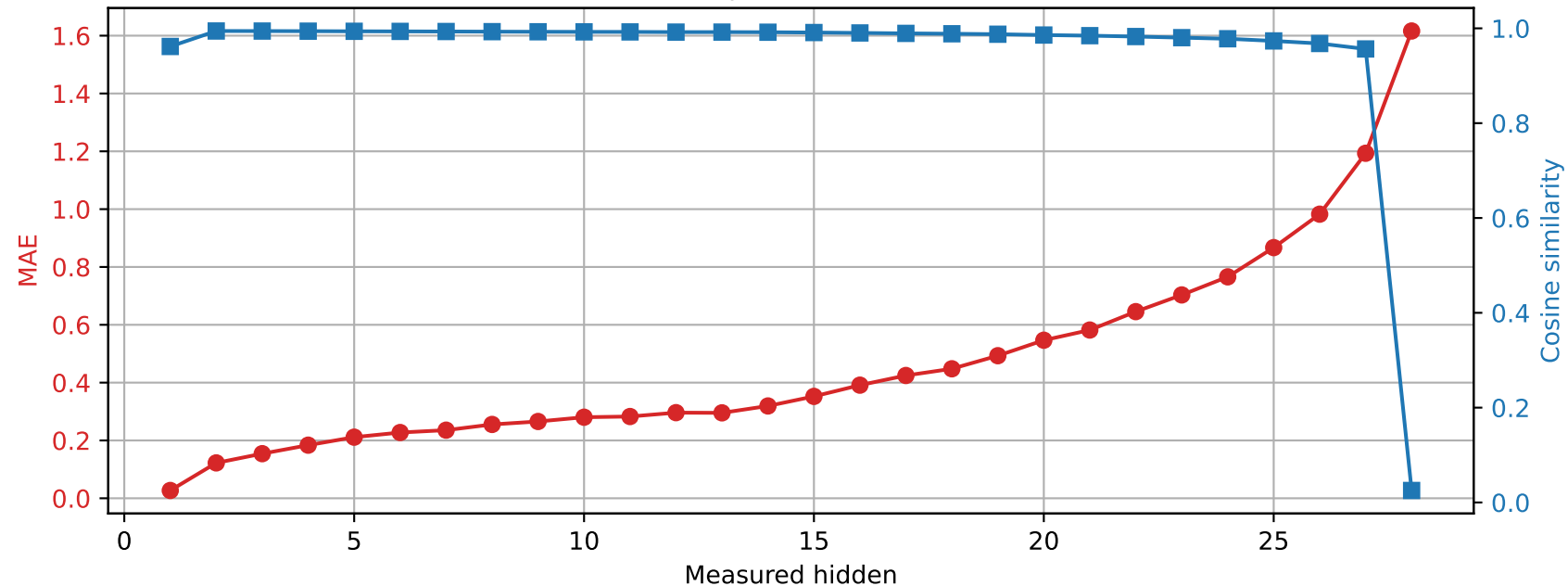
Llama-3.2-3B | Prompt 0 Spared layer 9 | Unquantized vs hybrid
