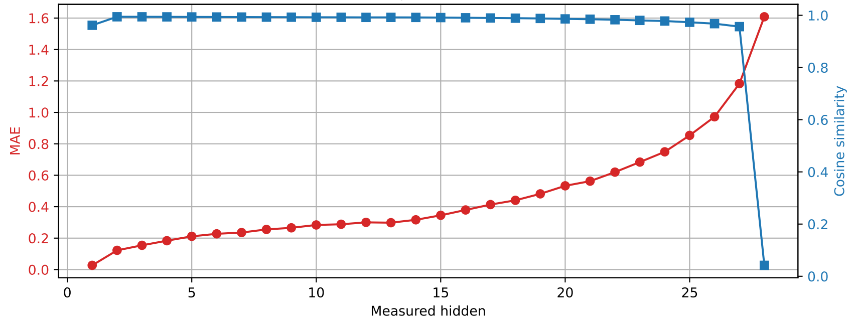
Llama-3.2-3B | Prompt 0 Spared layer 13 | Unquantized vs hybrid
