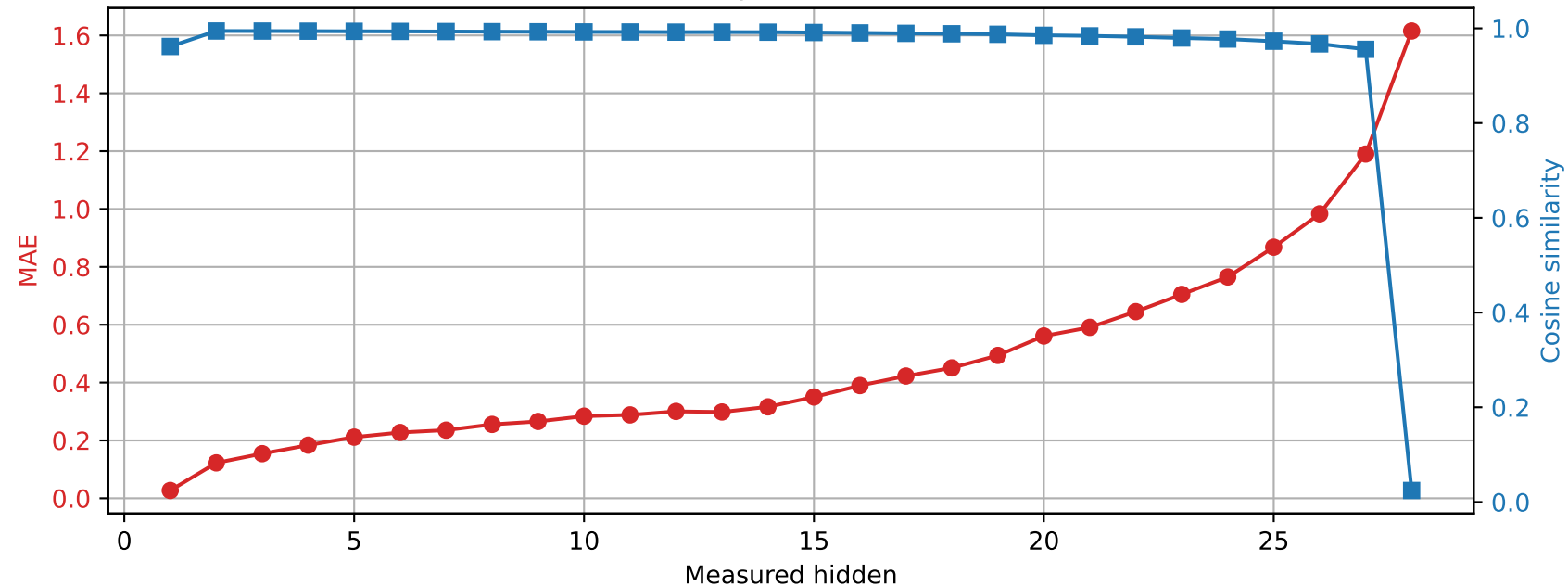
Llama-3.2-3B | Prompt 0 Spared layer 19 | Unquantized vs hybrid
