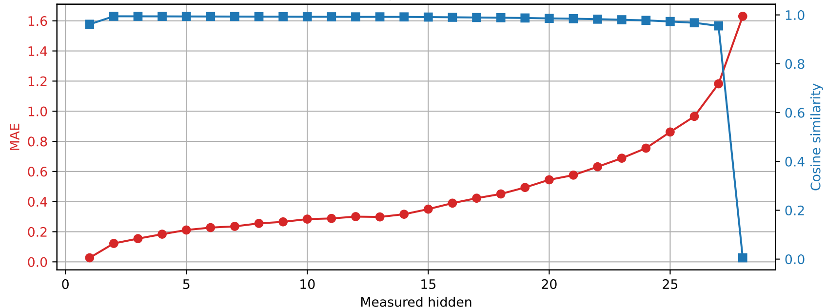
Llama-3.2-3B | Prompt 0 Spared layer 25 | Unquantized vs hybrid
