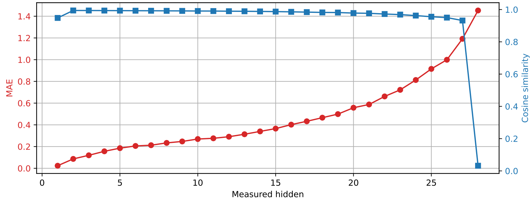
Llama-3.2-3B | Prompt 1 Spared layer 12 | Unquantized vs hybrid
