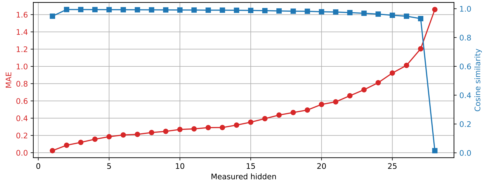
Llama-3.2-3B | Prompt 1 Spared layer 16 | Unquantized vs hybrid
