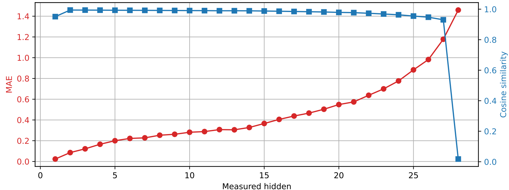
Llama-3.2-3B | Prompt 3 Spared layer 19 | Unquantized vs hybrid
