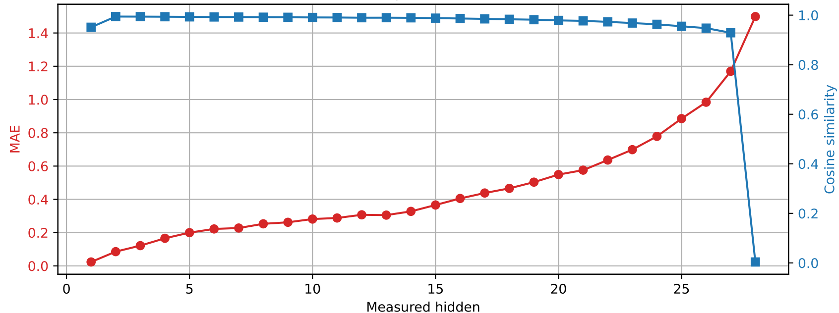
Llama-3.2-3B | Prompt 3 Spared layer 26 | Unquantized vs hybrid
