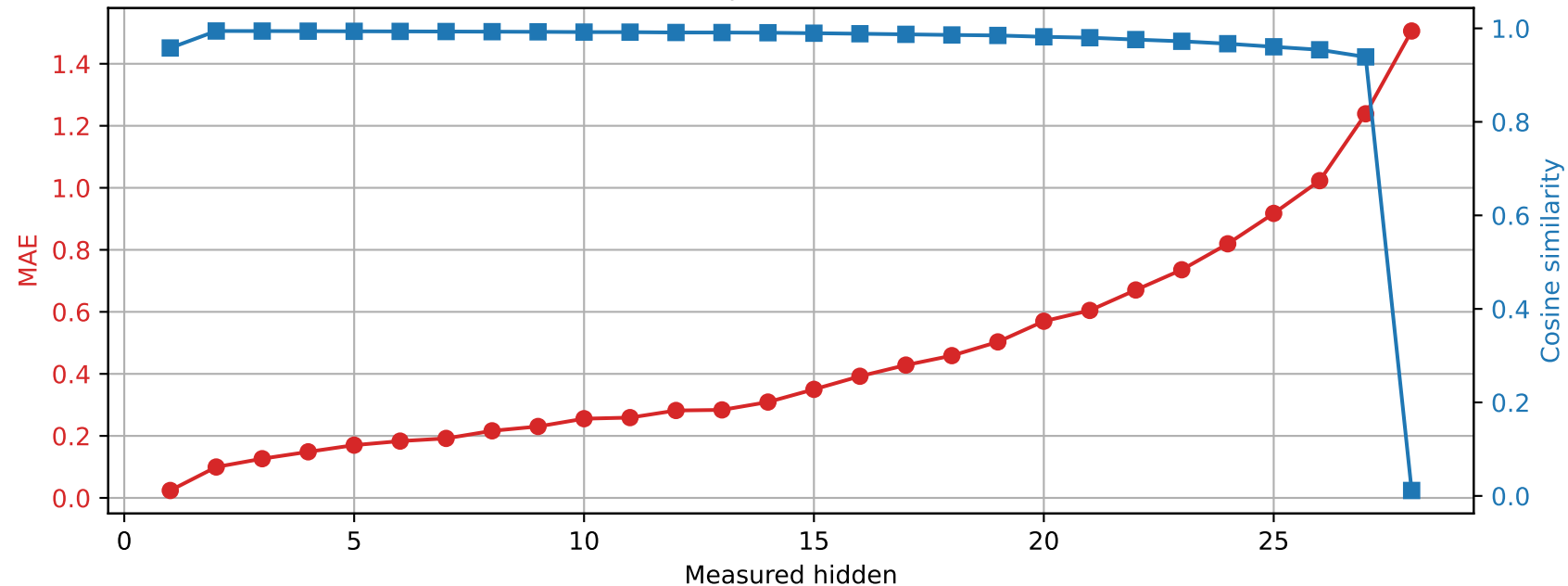
Llama-3.2-3B | Prompt 4 Spared layer 7 | Unquantized vs hybrid
